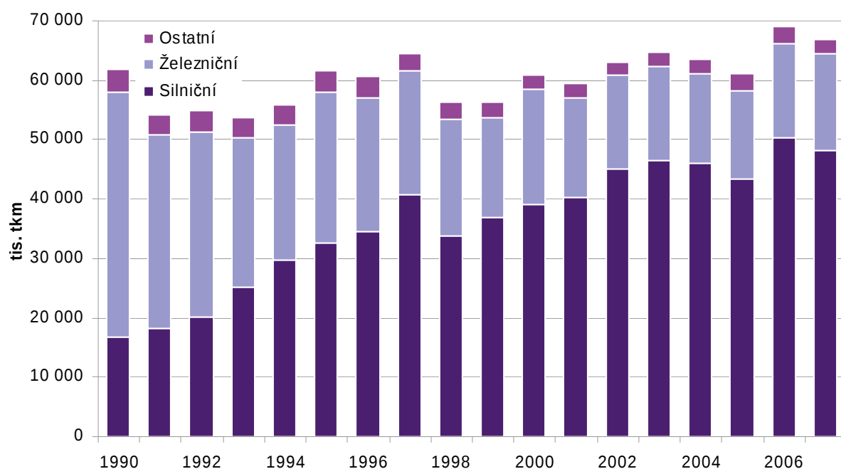
Graf III.5.2 Vývoj výkonů nákladní dopravy v letech 1989–2007
