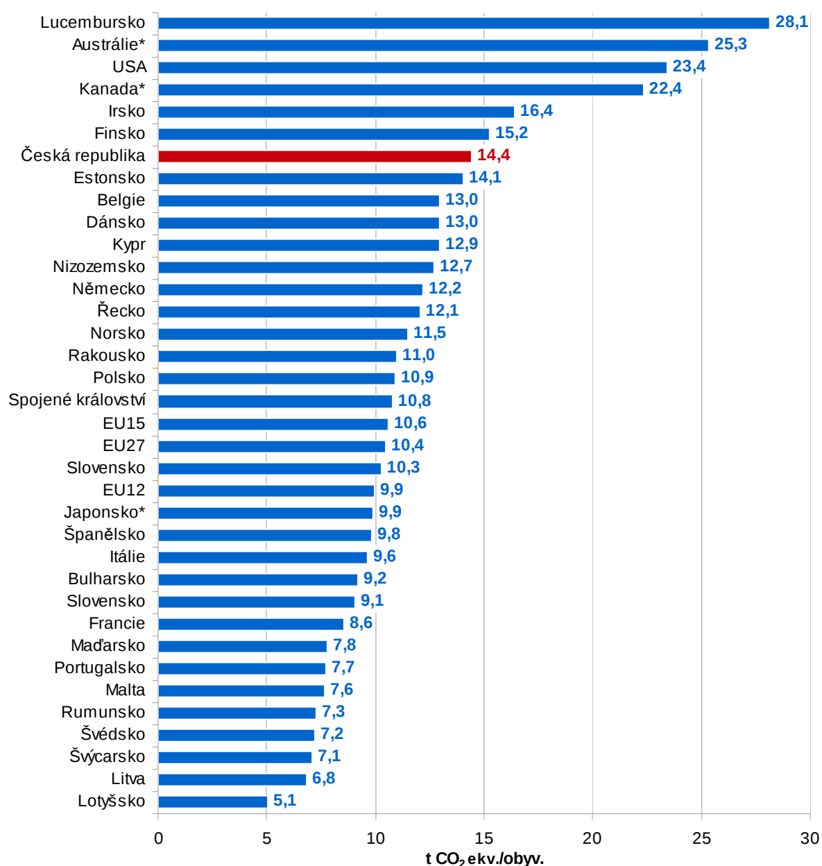
Graf I.1.14 Měrné emise CO 2 ekv. v EU27 a dalších státech v roce 2006
