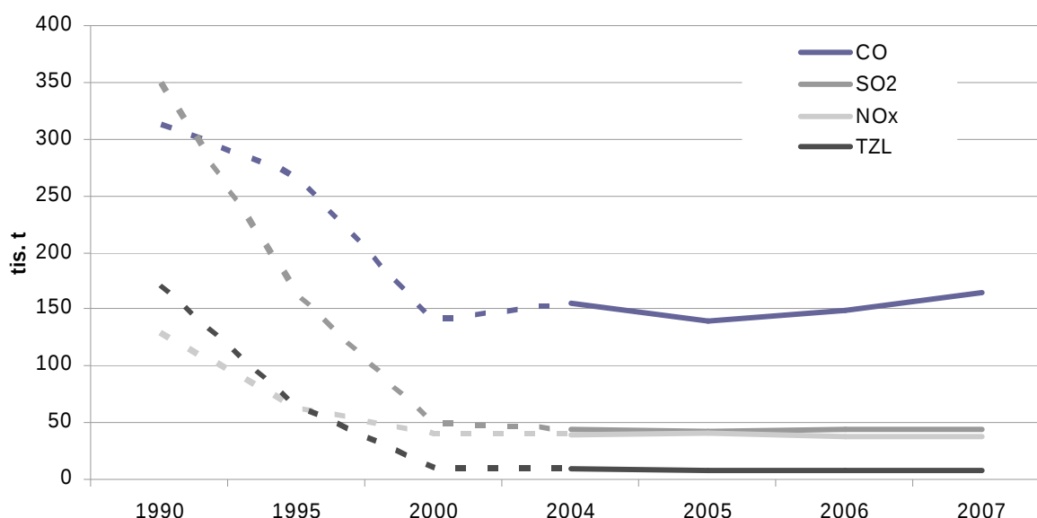
Graf III.4.7 Vývoj emisí znečišťujících látek ze zpracovatelského průmyslu
