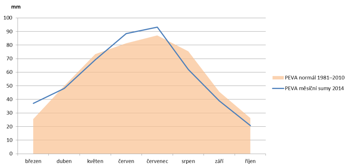
Graf 2: Měsíční úhrny potenciální evapotranspirace travního porostu (PEVA) v období březen–říjen roku 2014 a průměrná hodnota měsíčních úhrnů PEVA v normálovém období 1981–2010 [mm]
