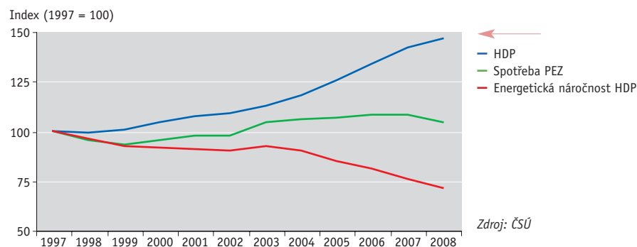
Graf 1 → Energetická náročnost HDP ČR [index, 1997 = 100], 1997–2008
