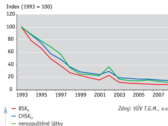
Graf 1 → Relativní vyjádření vypouštěného znečištění v ukazatelích BSK 5 , CHSK Cr a NL [index, 1993 = 100], 1993–2008
