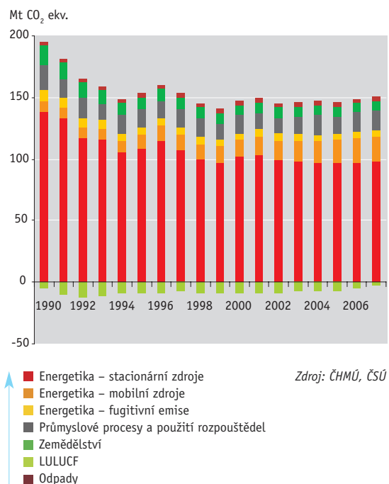
Graf 3 → Vývoj emisí skleníkových plynů v ČR v sektorovém členění [Mt CO 2 ekv.], 1990–2007
