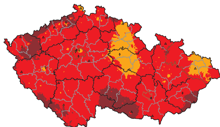
Obr. 1 → Pole hodnot indexu AOT40, průměr za 5 let [μg.m -3 .h], 2004–2008
