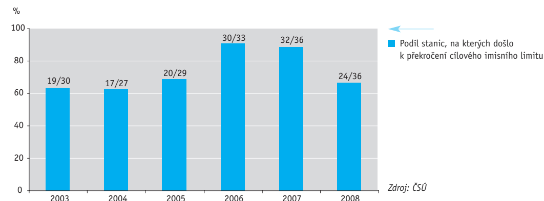
Graf 1 → Podíl stanic, na kterých došlo k překročení cílového imisního limitu vyjádřeného jako AOT40 (průměr za 5 let) pro ochranu vegetace [%], 2003–2008
