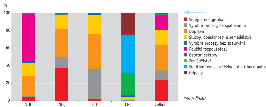
Graf 2 → Zdroje emisí prekurzorů ozonu v ČR [%], 2007
