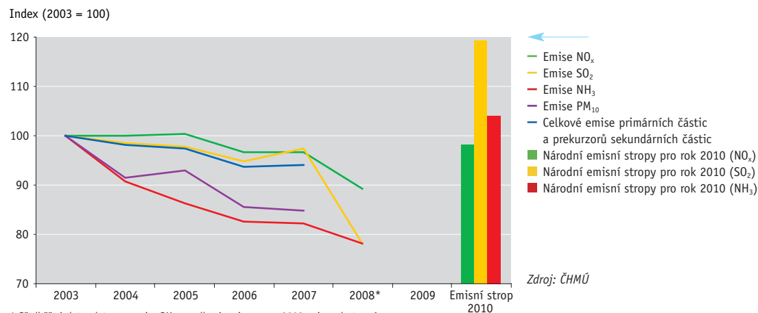
Graf 1 → Vývoj emisí primárních částic a prekurzorů sekundárních částic v ČR, 2003–2008* a úroveň národních emisních stropů (pro NO_x , SO_2 a NH_3 ) pro rok 2010 [index, 2003 = 100]
