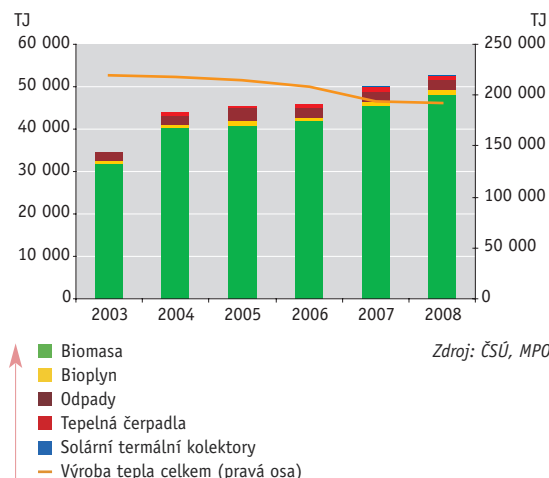
Graf 3 → Výroba tepla z obnovitelných zdrojů energie, celková výroba tepla v ČR [TJ], 2003–2008
