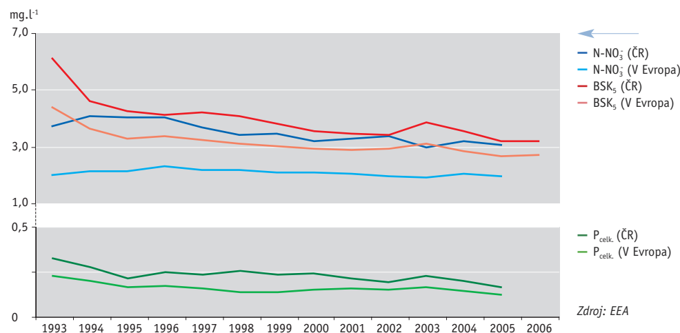
Graf 4 → Srovnání průměrných hodnot koncentrací ukazatelů znečištění v tocích ČR a východní Evropy [mg.l -1 ], 1993–2006
