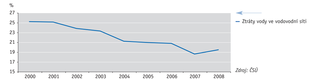
Graf 3 → Ztráty vody ve vodovodní síti v ČR [%], 2000–2008
