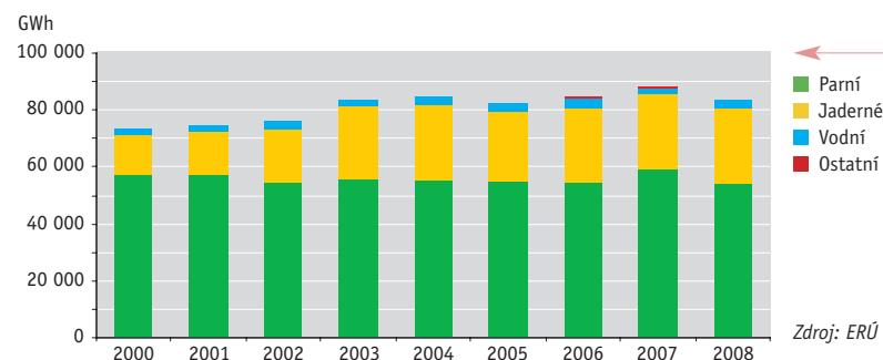
Graf 1 → Výroba elektřiny podle druhu elektráren v ČR [GWh], 2000–2008
