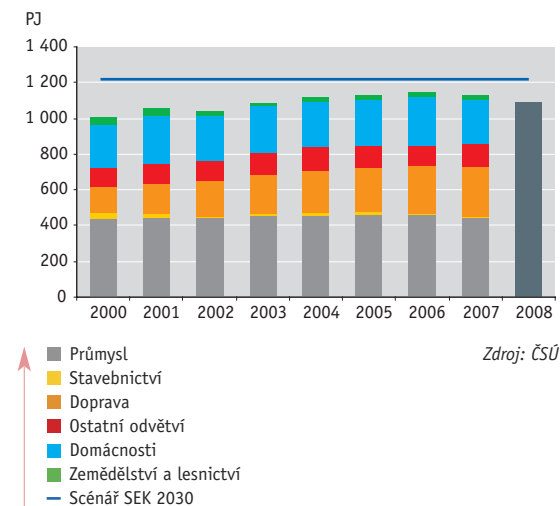
Graf 2 → Vývoj konečné spotřeby energie dle odvětví v ČR [PJ], 2000–2008
