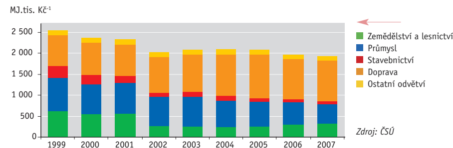
Graf 3 → Vývoj energetické náročnosti dle sektorového členění vyjádřený podílem konečné spotřeby energie sektoru a hrubé přidané hodnoty sektoru ČR [MJ.tis. Kč -1 ], 1999–2007
