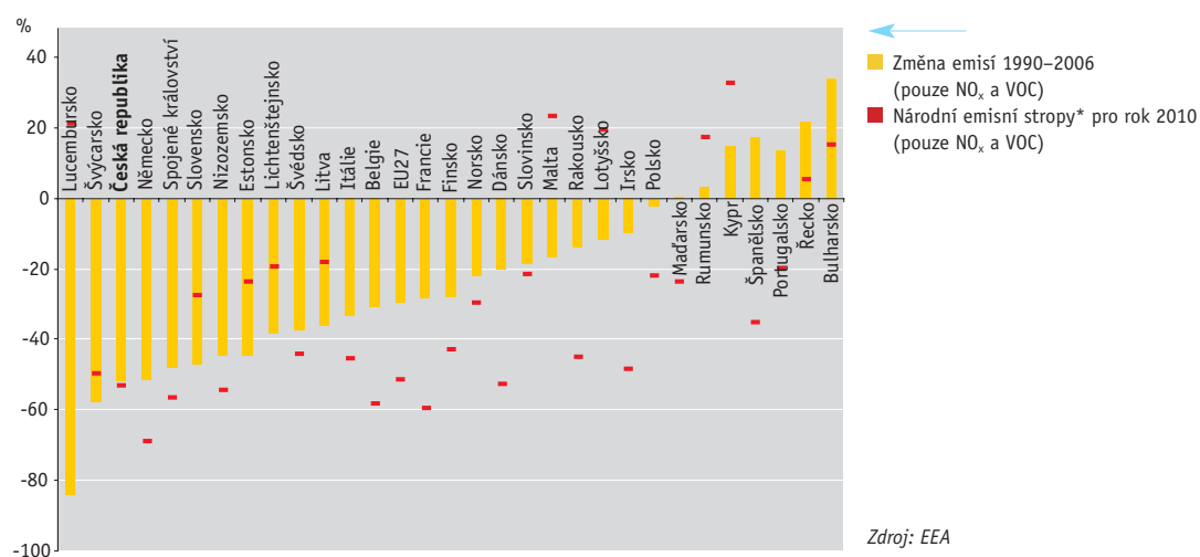
Graf 3 → Vzdálenost úrovně emisí prekurzorů ozonu (pouze NO x a VOC) v roce 2006 od jednotlivých národních emisních stropů pro rok 2010 ve vybraných státech Evropy [%]
