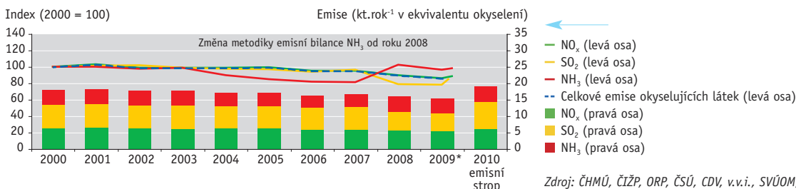
Graf 1 → Vývoj celkových emisí oxyselujících látek v ČR, 2000–2009*, a úroveň národních emisních stropů pro rok 2010 [index, 2000 = 100]; [ \text{kt.rok}^{-1} v ekvivalentu oxyselení]
