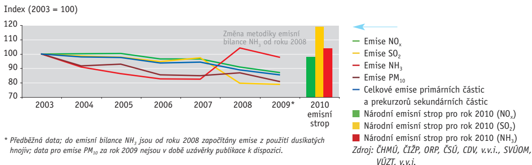
Graf 1 → Vývoj emisí primárních částic a prekursorů sekundárních částic v ČR, 2003–2009*, a úroveň národních emisních stropů (pro \text{NO}_x , \text{SO}_2 a \text{NH}_3 ) pro rok 2010 [index, 2003 = 100]
