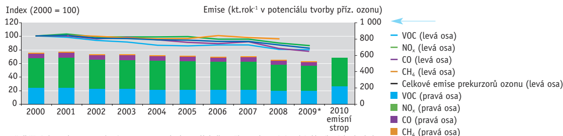
Graf 1 → Vývoj celkových emisí prekurzorů ozonu v ČR, 2000–2009*, a úroveň národních emisních stropů (pro VOC a \text{NO}_x ) pro rok 2010 [index, 2000 = 100]; [ \text{kt.rok}^{-1} v potenciálu tvorby přízemního ozonu]
