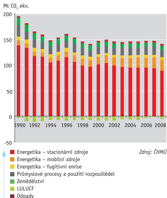
Graf 3 → Vývoj emisí skleníkových plynů v ČR v sektorovém členění [Mt CO 2 ekv.], 1990–2008
