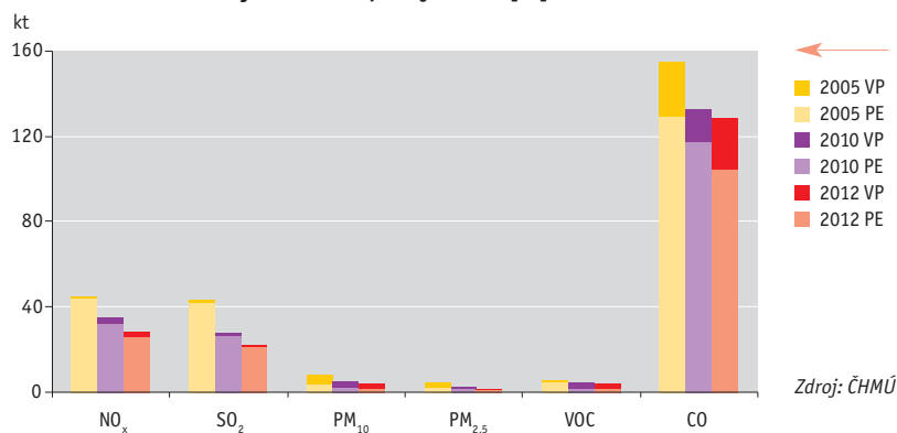
Graf 3 → Emise znečišťujících látek z průmyslu v ČR [kt], 2005, 2010, 2012
