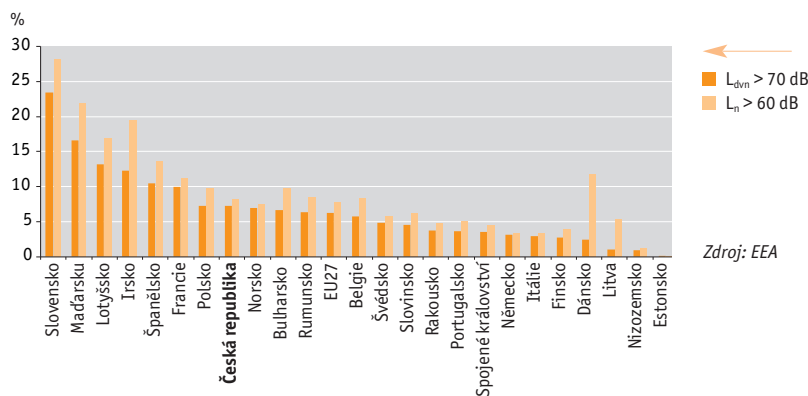
Graf 4 → Hluková zátěž ze silniční dopravy v aglomeracích nad 250 tis. obyvatel, přesahující mezní hodnoty dle legislativy ČR pro celodenní obtěžování hlukem ( L_{dn} ) a noční hlukovou zátěž ( L_n ) [% exponovaných obyvatel aglomerací], 2009
