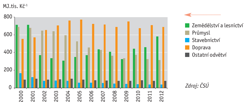
Graf 3 → Vývoj energetické náročnosti dle sektorového členění vyjádřený podílem konečné spotřeby energie sektoru a hrubé přidané hodnoty sektoru v ČR [MJ.tis. Kč -1 ], 2000–2012
