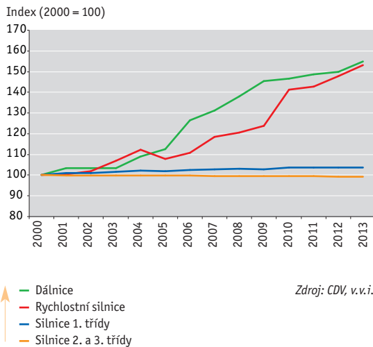
Graf 4 → Vývoj silniční a dálniční sítě v ČR [index, 2000 = 100], 2000–2013
