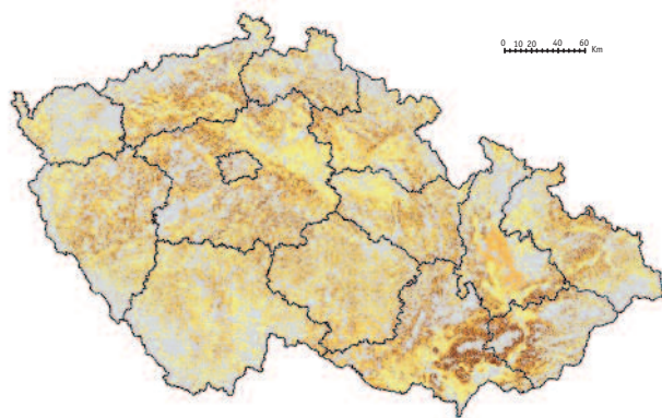
Obr. 1 → Potenciální ohroženost zemědělské půdy vodní erozí v ČR, vyjádřená dlouhodobým průměrným smyvem půdy G [t.ha -1 .rok -1 ], 2013
