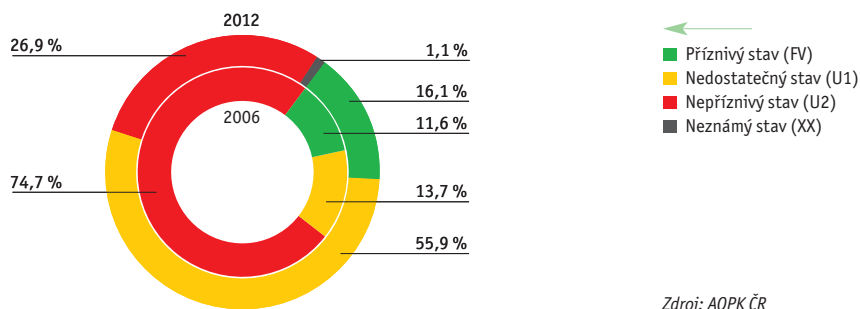
Graf 1 → Vyhodnocení stavu evropsky významných typů přírodních stanovišť v ČR [%], 2000–2006, 2007–2012
