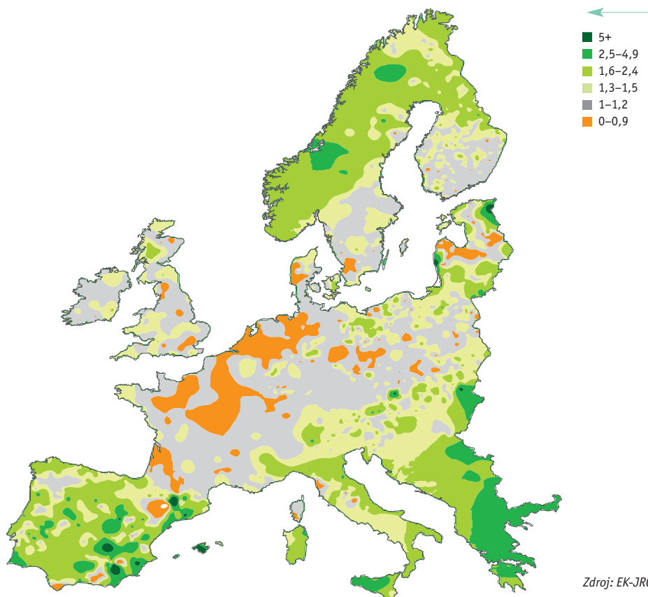
Obr. 1 → Evropské lesní oblasti podle hodnoty C/N indexu, 2008
