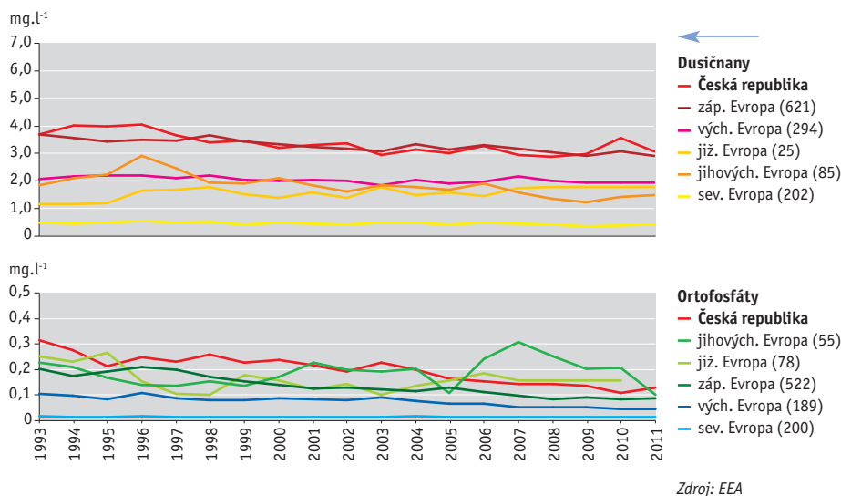
Graf 4 → Znečištění nutrienty v tocích ČR a evropských georegionů [ \text{mg} \cdot \text{l}^{-1} ], 1993–2011
