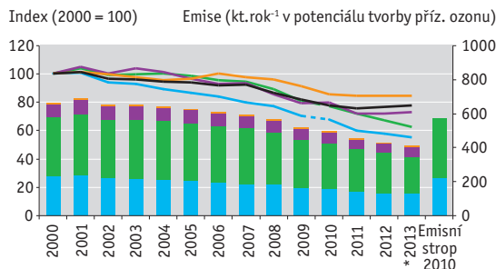
Graf 1 → Vývoj celkových emisí prekurzorů ozonu v ČR a úroveň národních emisních stropů (pro VOC a NO x ) pro rok 2010 [index, 2000 = 100]; [kt.rok -1 v potenciálu tvorby přízemního ozonu], 2000–2013
