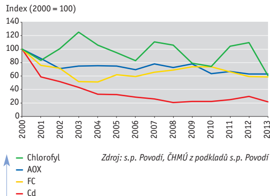
Graf 2 → Vývoj koncentrací ukazatelů znečištění ve vodních tocích [index, 2000 = 100], 2000–2013
