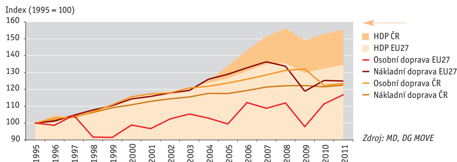
Graf 1 → Vývoj přepravních výkonů osobní a nákladní dopravy a HDP v ČR a v EU27 [index, 1995 = 100], 1995–2011
