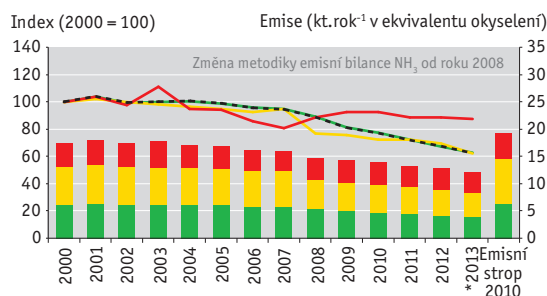
Graf 1 → Vývoj celkových emisí oxyselujících látek v ČR a úroveň národních emisních stropů pro rok 2010 [index, 2000 = 100]; [kt.rok -1 v ekvivalentu oxyselení], 2000–2013
