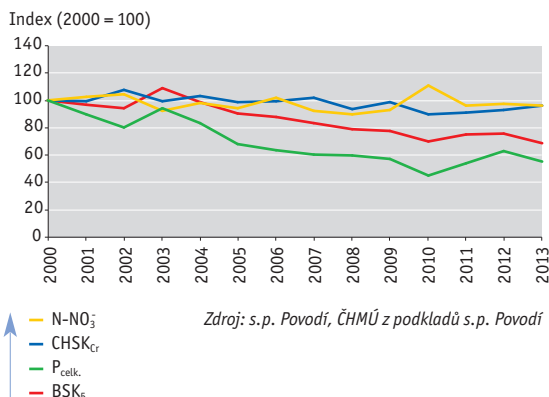
Graf 1 → Vývoj koncentrací ukazatelů znečištění ve vodních tocích [index, 2000 = 100], 2000–2013
