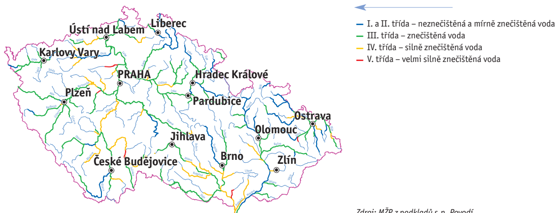
Obr. 1 → Jakost vody v tocích ČR, 2012–2013
