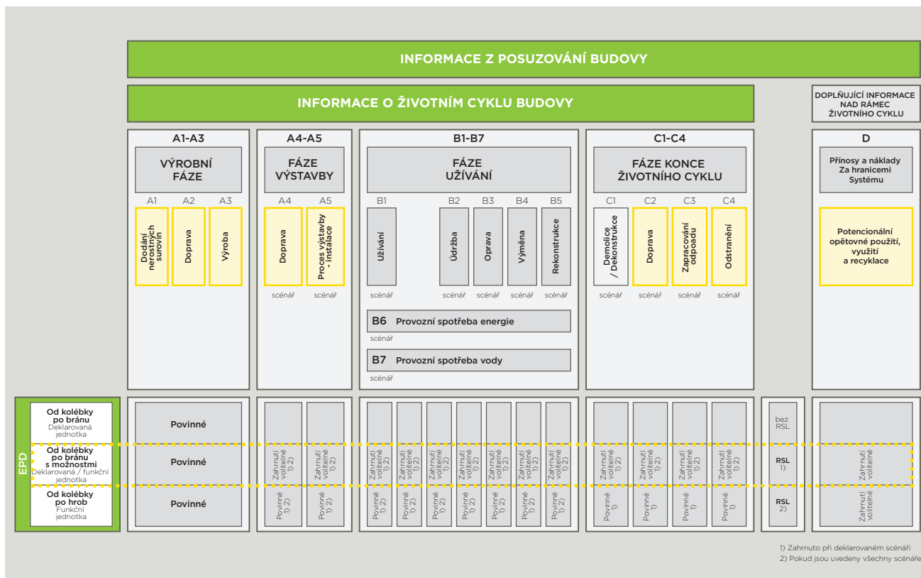
Obr. 3 – Započítané fáze životního cyklu (ČSN EN 15804+A1); vliv výroby ve fázi B1-B7 bude započítán až na úrovni konstrukce, budovy
