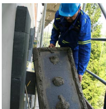
Obr. 1 – Příklad použití výrobku Isover EPS GreyWall
