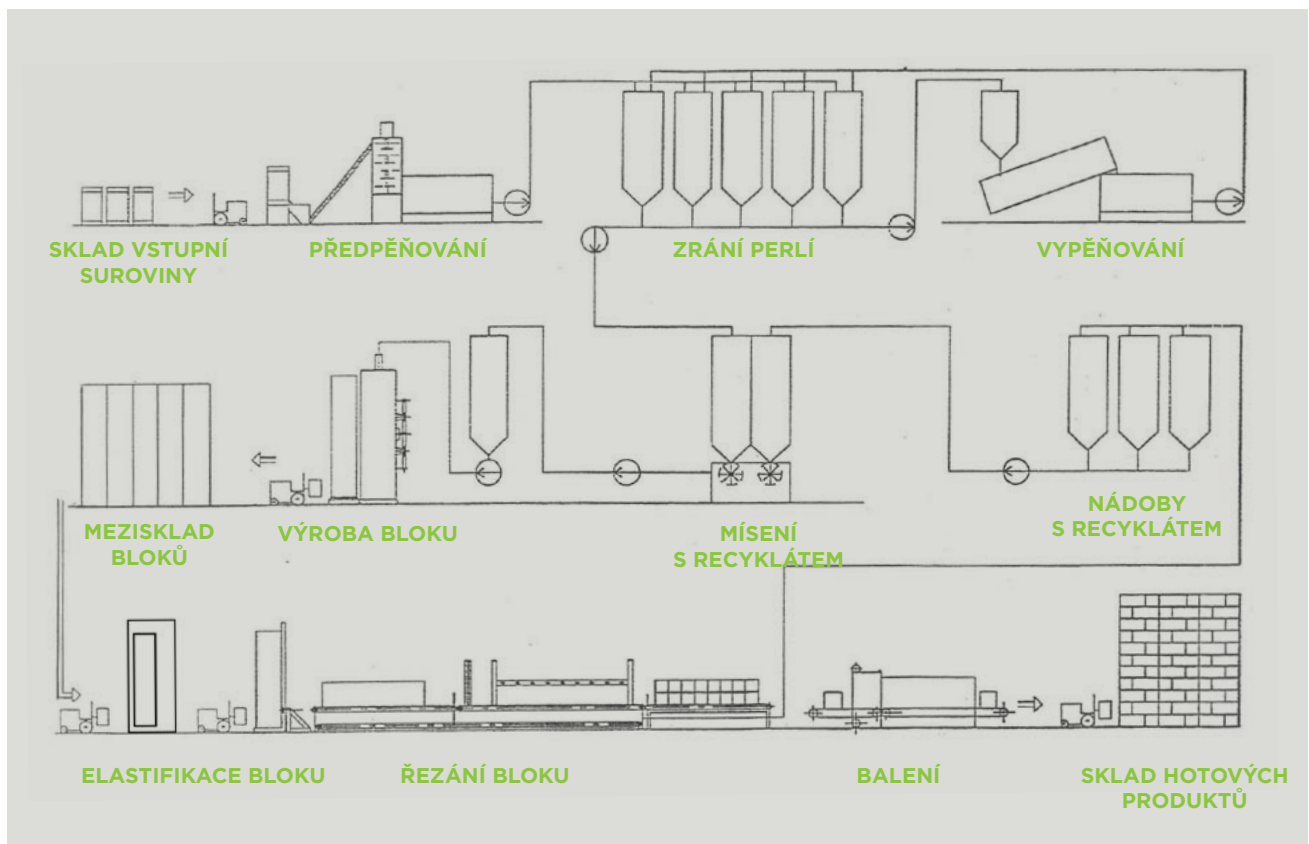
Obr. 3 – Schéma výroby elastifikovaného pěnového polystyrenu
