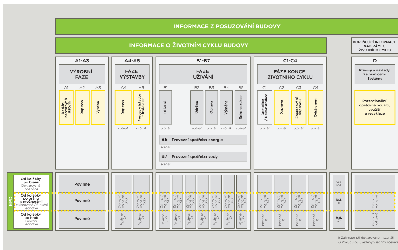
Obr. 3 – Započítané fáze životního cyklu (ČSN EN 15804+A1); vliv výrobku ve fázi B1-B7 bude započítán až na úrovni konstrukce, budovy
