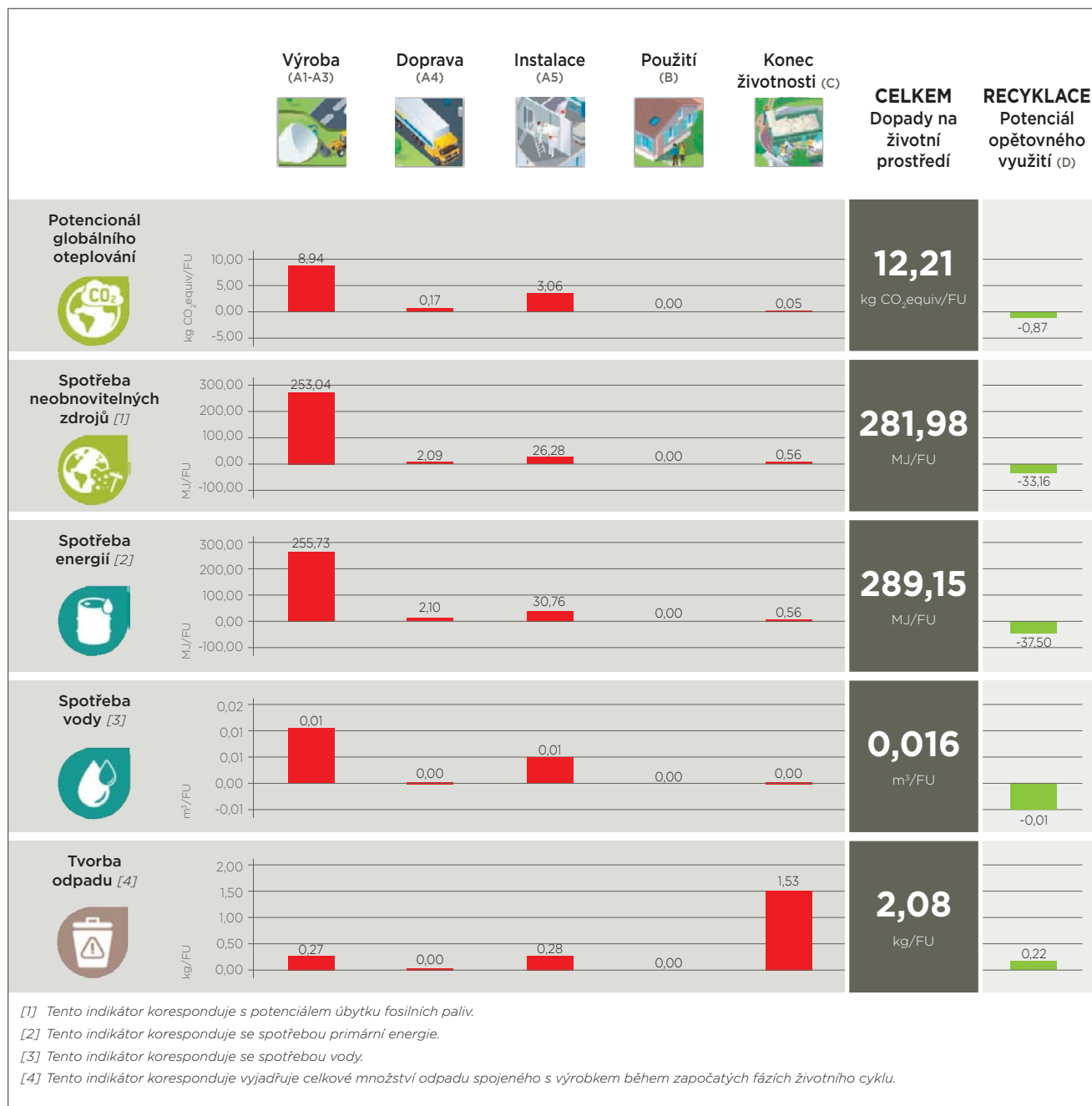
Obr. 5 – Interpretace výsledků LCA dle SG PCR
