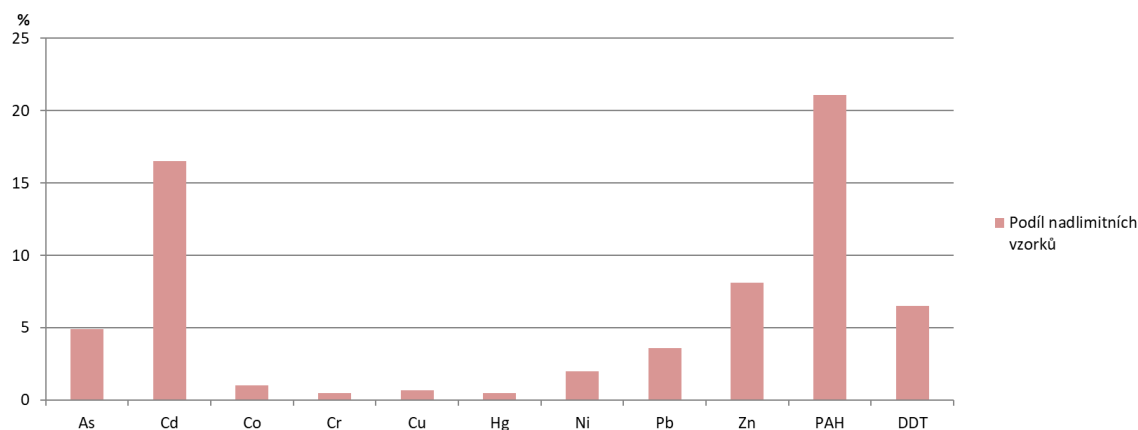
Podíl vzorků rybníčních a říčních sedimentů překračujících limitní hodnoty v ČR [%], 1995–2018
