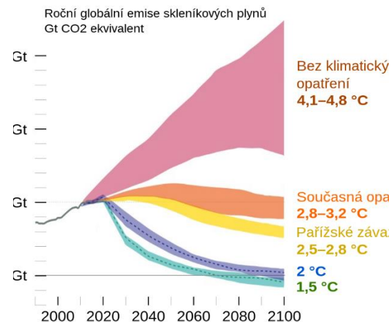
Scénáře globálních emisí skleníkových plynů
